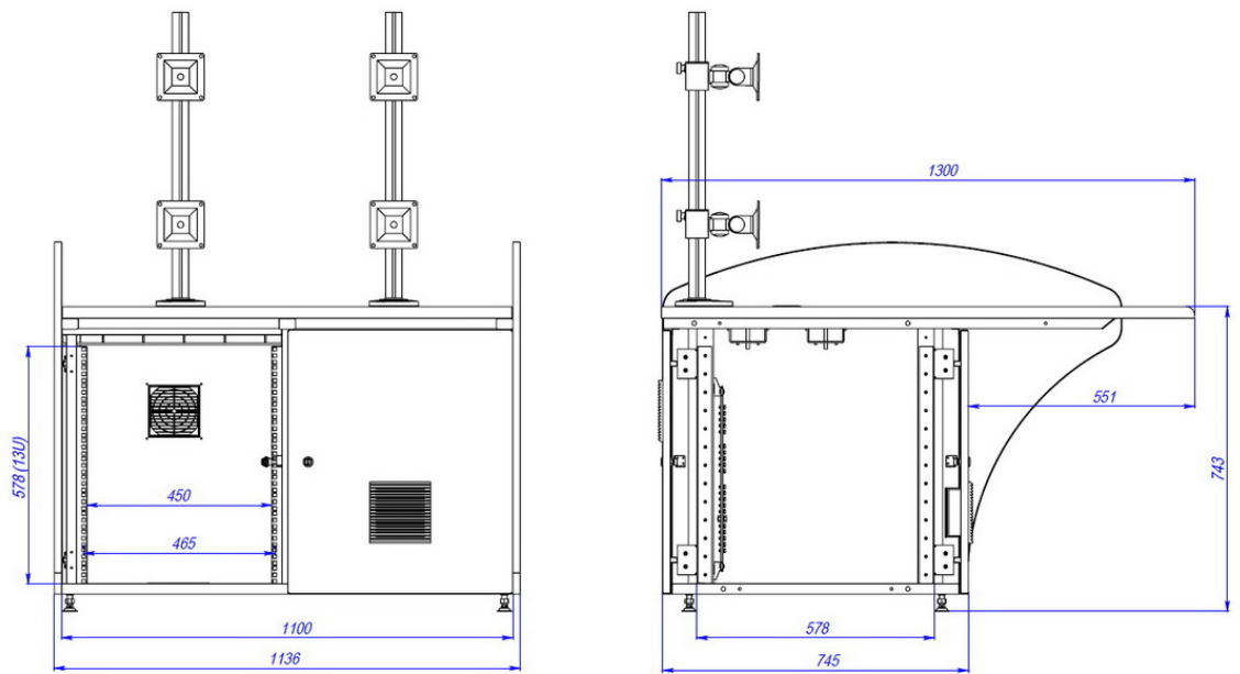
Рис. 2. Стол оператора
